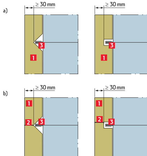
Karimák szigetelési módjai
