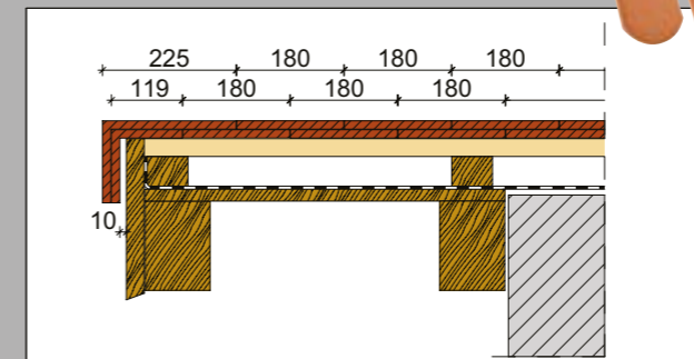
Oromszegély 3/4 és 5/4 szegélycserepekkel
