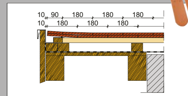
Oromszegély 1/2 és 1/1 hódfarkú cserepekkel
