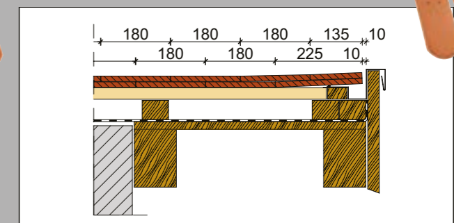
Oromszegély 3/4 és 5/4 hódfarkú cserepekkel
