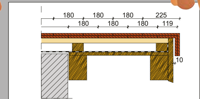
Oromszegély 3/4 és 5/4 szegélycserepekkel
