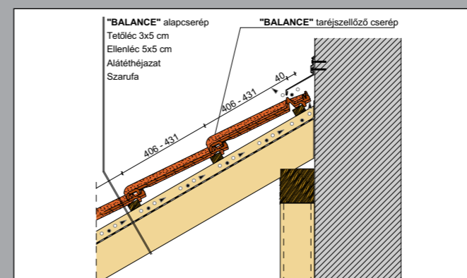
Falszegély kialakítás
