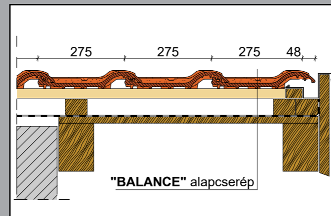
Oromszegély, alapcseréppel
