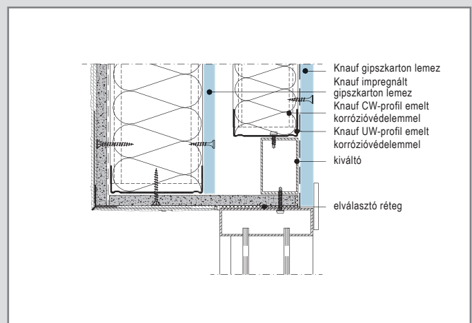
W387E-FE-VO2 Szemöldök csatlakozás 2
