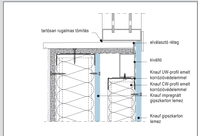
W387E-FE-VU2 Párkány kialakítás 2
