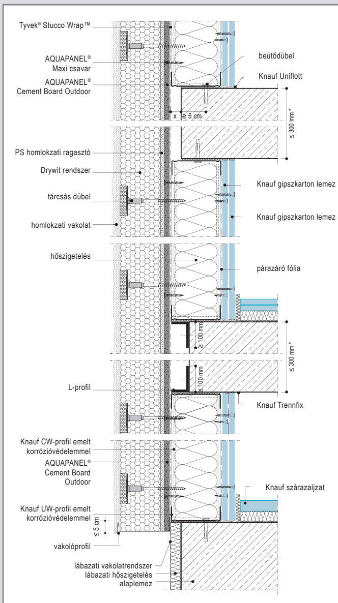
W384E-V-ETICS1 Metszet
