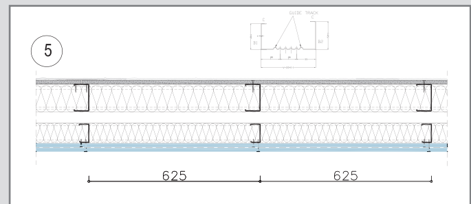
05. Perforált profilos szerkezet
