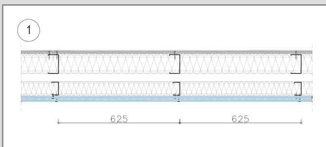
01. Alapszerkezet
