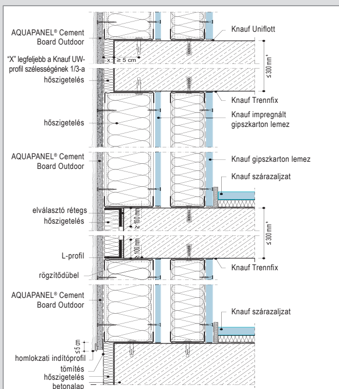
W387E-V1 Metszet
