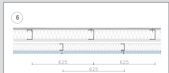
06. Váltott profilelhelyezésű kettős váz hőszigeteléssel
