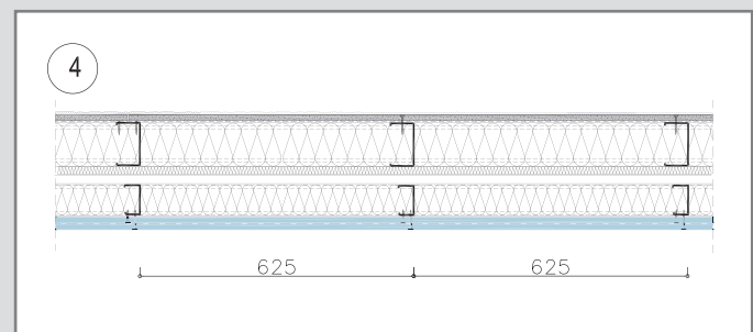
04. Kettős váz kettős hőszigeteléssel
