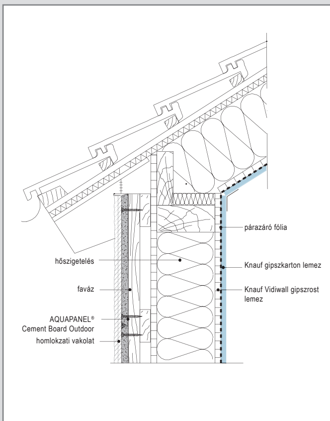
W681-DA-V1 Térfal kialakítás
