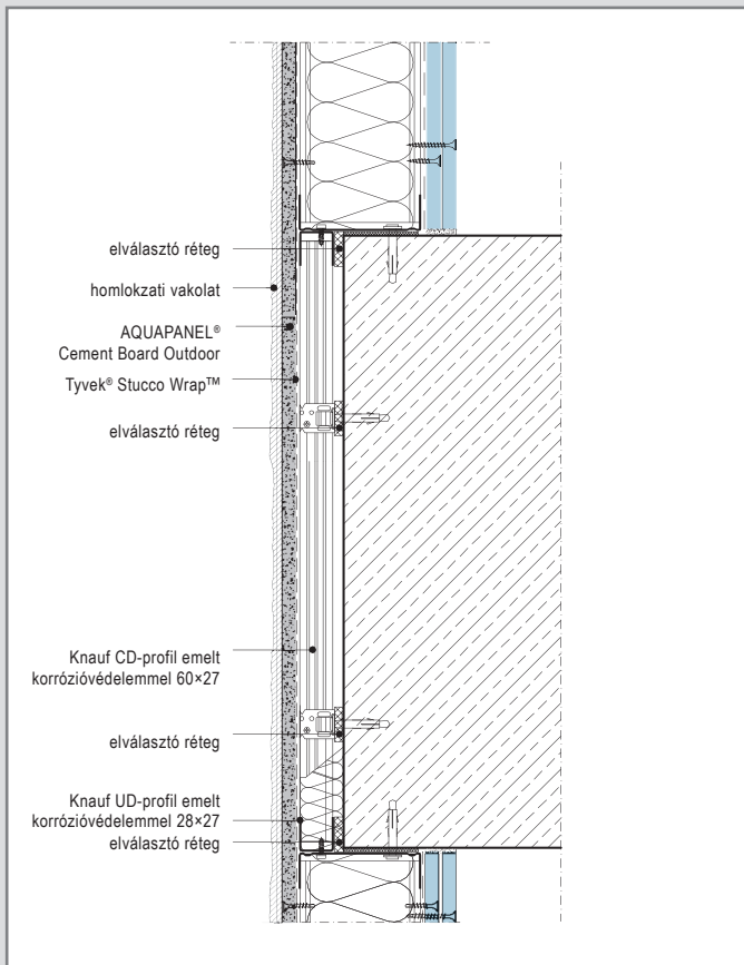
W384E-VM1 Födémsegély kialakítás
