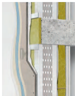
Födémre állított szerkezet perforált profilú vázzal
