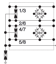
Kapcsolási rajz
