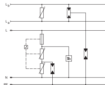
Kapcsolási rajz
