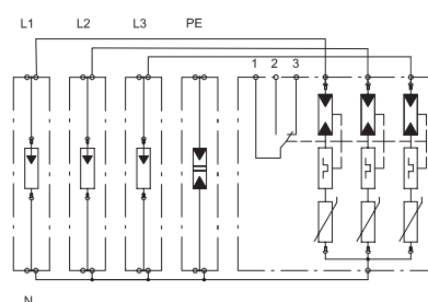
Kapcsolási rajz
