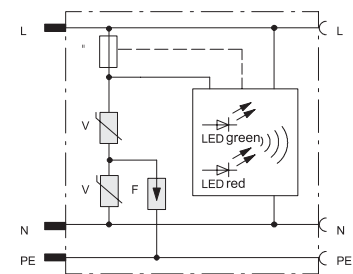
Kapcsolási rajz
