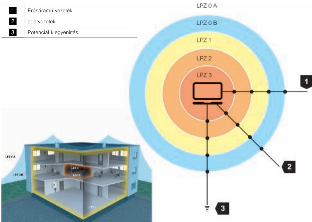
Védelmi elv a villámzédelmi zónakoncepció alapján
