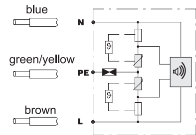
Kapcsolási rajz
