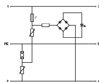
Kapcsolási rajz
