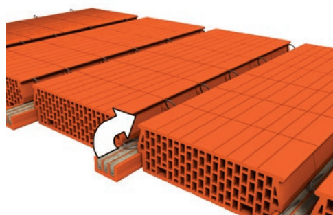
9 A kengyelek felhajlítása
