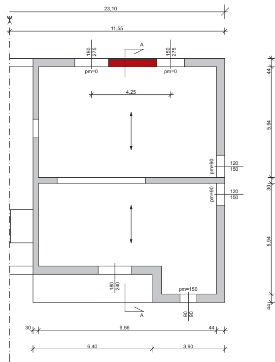
Sematicus alaprajz (földszint + emelet)
