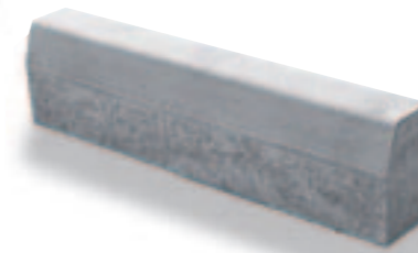
Kiemelt útszegély kopóréteggel Méret: 100 x 25 x 15 cm
