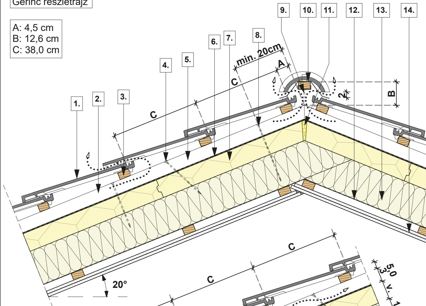
Eresz részletrajz
