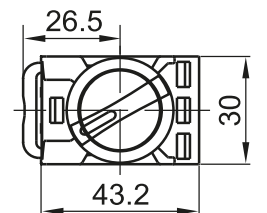
Háromállású rugóvisszatérítéses
