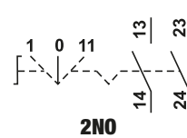
Háromállású rugóvisszatérítéses
